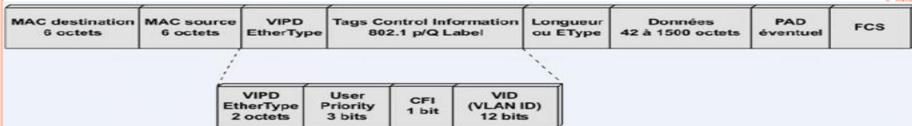
Trame MAC des réseaux de type 802.3 + Tag
